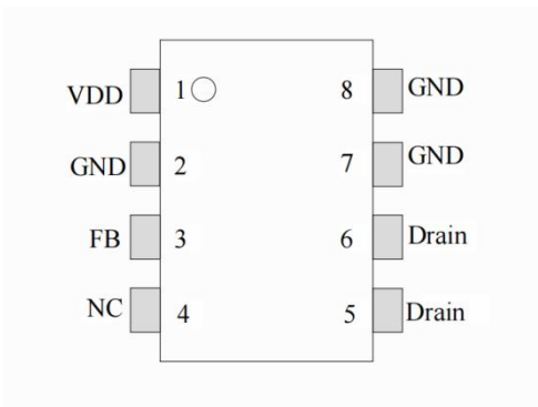
SOP-8俯视图
